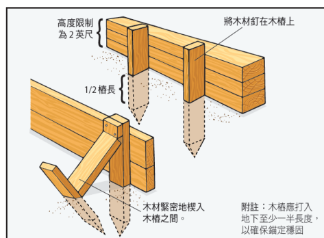
木製導流牆
