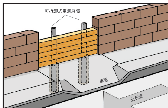
圖 20 - 可拆卸式車道屏障（單桿）
