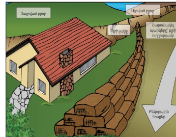
Նկ. 7 ԱՂԲԻ ՀԵՌԱՑՈՒՄԸ ՇԵՆՔԻՑ
