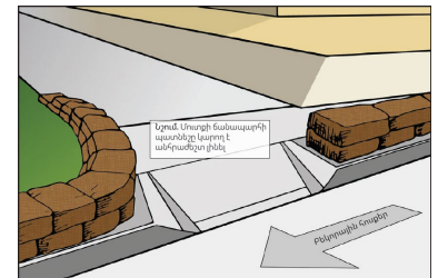
Նկ. 8 ԲԵԿՈՐՆԵՐԻ ՎԵՐԱՀԱՄԱԿՈՒՄ ԿԱՄ ՓՈԹՈՐԿԱՅԻՆ ՀՈՍՔԵՐԸ ՓՈՂՈՑՆԵՐՈՒՄ
